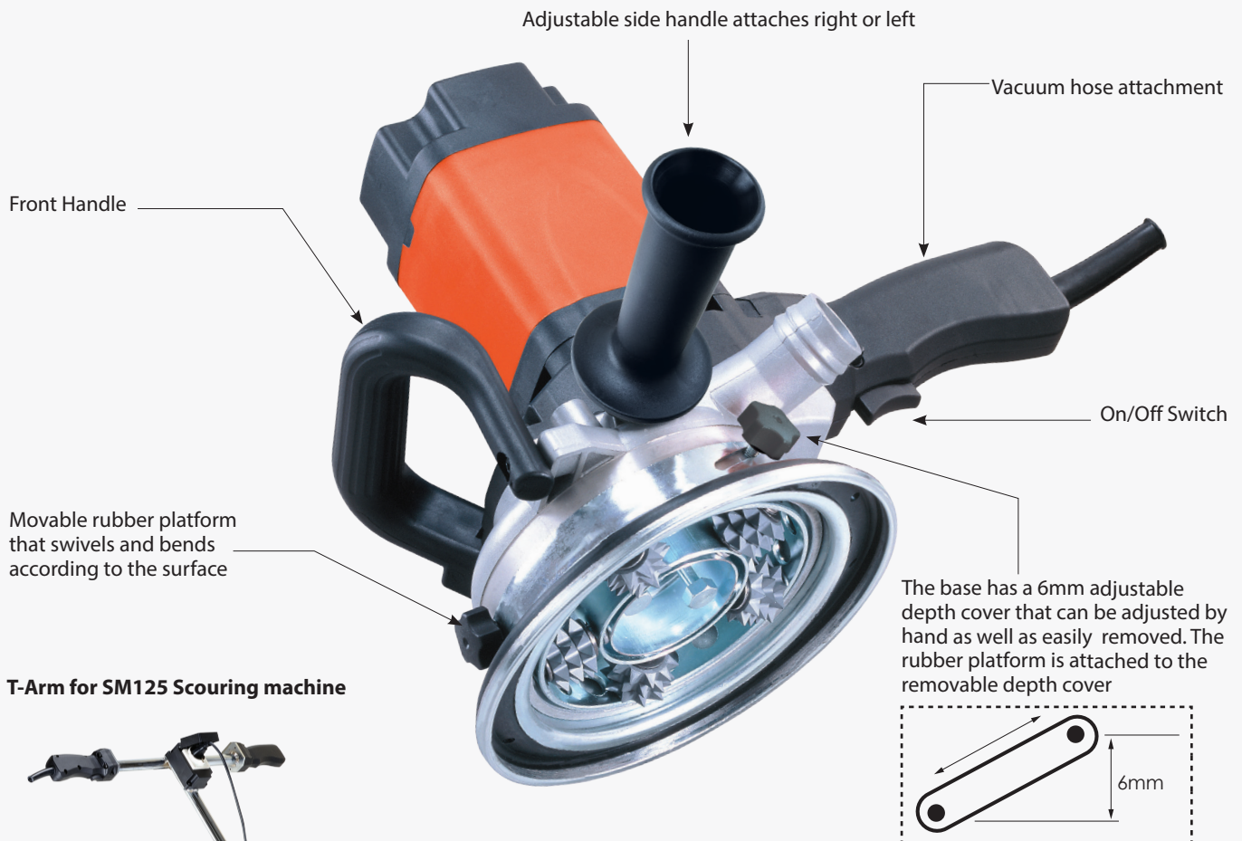
T-Arm (Optional)
